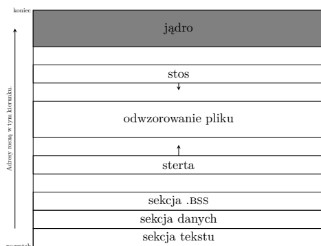
Rysunek 1: Uproszczony model przestrzeni adresowej w Linuksie
