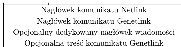
Rysunek 3: Format komunikatu Genetlink (na podstawie https://wiki.linuxfoundation.org/networking/generic_netlink_howto )
