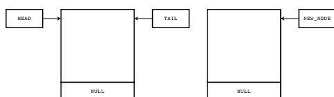
Przed wykonaniem 10 wiersza funkcji enqueue()
