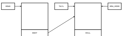
Po wykonaniu 11 wiersza funkcji enqueue()
