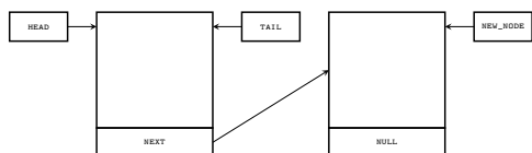
Po wykonaniu 10 wiersza funkcji enqueue()
