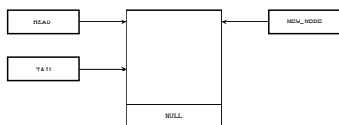
Kolejka po wykonaniu 8 wiersza funkcji enqueue()
