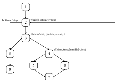
Rysunek: Graf przepływu sterowania
