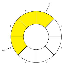
Częściowo wypełniona kolejka FIFO
