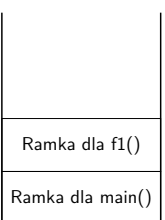
Stos po zakończeniu funkcji f2()
